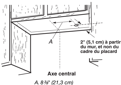
A. 8 3/8" (21,3 cm)
